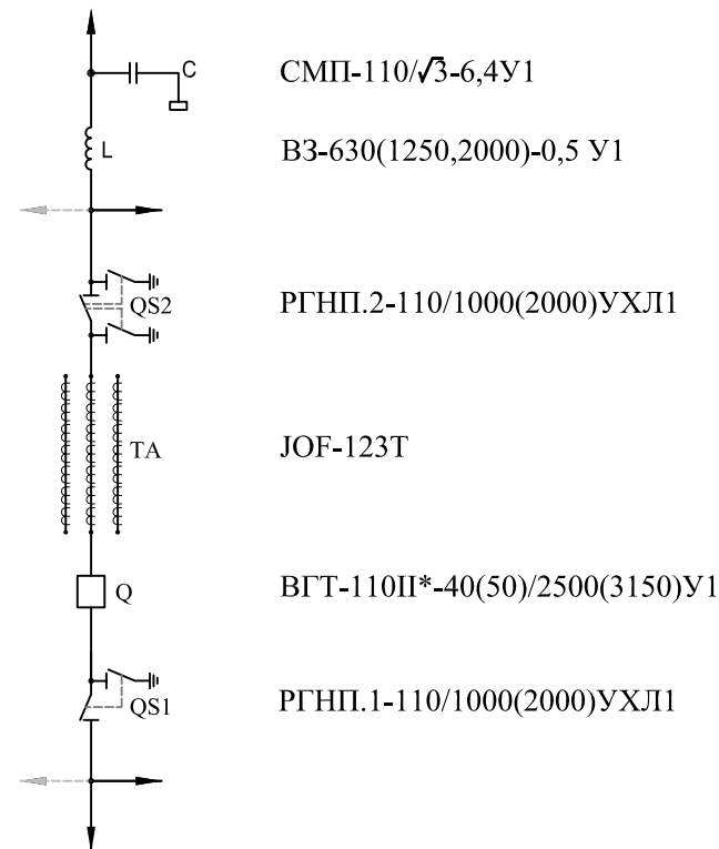
Принципиальная схема
