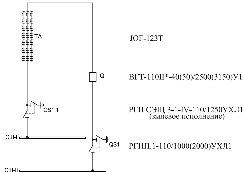
Принципиальная схема
